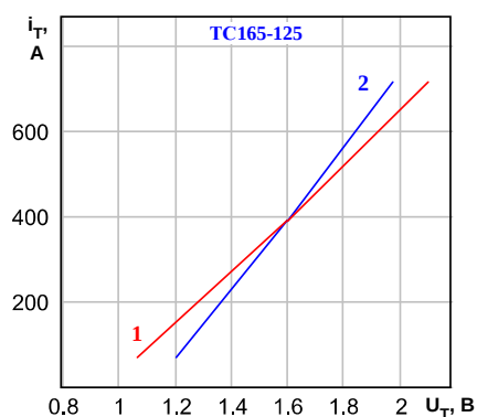
Рисунок 1: Пределы вольтамперные характеристики при максимально допустимой температуре перехода T_{jm} (1) и температуре T_j=25^\circ\text{C} (2), I_T=1,41 I_{TRMSM} .
