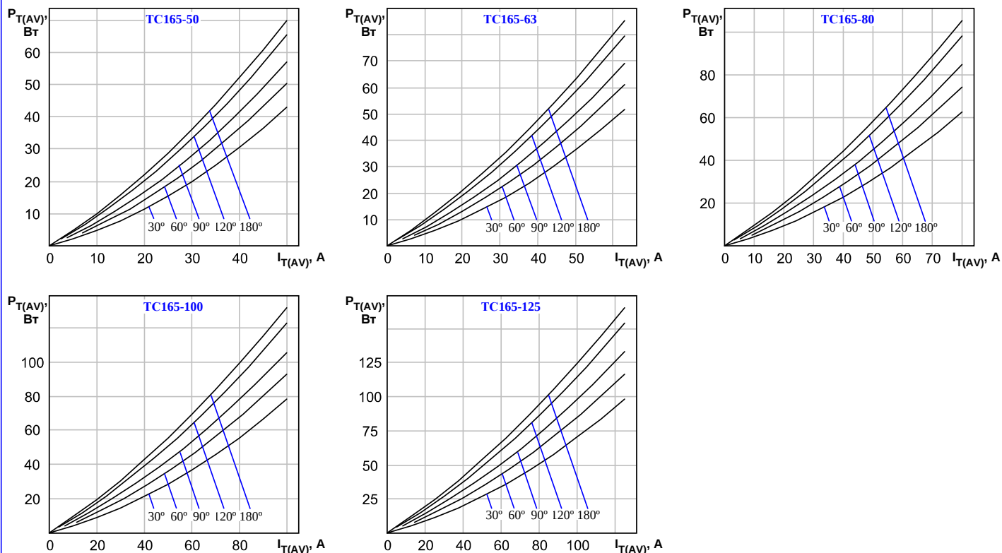
Рисунок 4: Зависимость средней мощности потерь P_{T(AV)} от действующего значения тока I_{T(ARMS)} в открытом состоянии синусоидальной формы частотой 50 Гц при различных углах проводимости.
