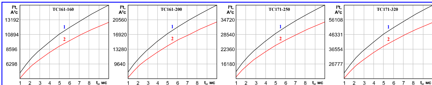
Рисунок 6: Зависимость защитного показателя I^2t от длительности импульса тока t_i при исходной температуре структуры T_j=25^\circ\text{C} (1) и максимально допустимой температуре перехода T_{jm} (2).
