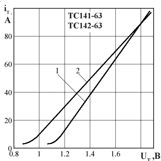
Рисунок 1 - Предельная вольтамперная характеристика в открытом состоянии при температуре перехода 25 °C (1) и максимальной температуре перехода T_{jm} (2)
