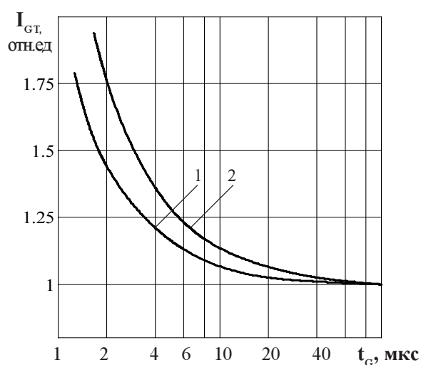
Рисунок 10 - Зависимость отпирющего импульсного тока управления I_{GT} от длительности управляющего импульса t_g при температуре перехода T_j = 25\text{ }^{\circ}\text{C} (1), T_{jmin} = \text{минус } 50\text{ }^{\circ}\text{C} (2) и напряжения в закрытом состоянии U_D = 12\text{ В} .
