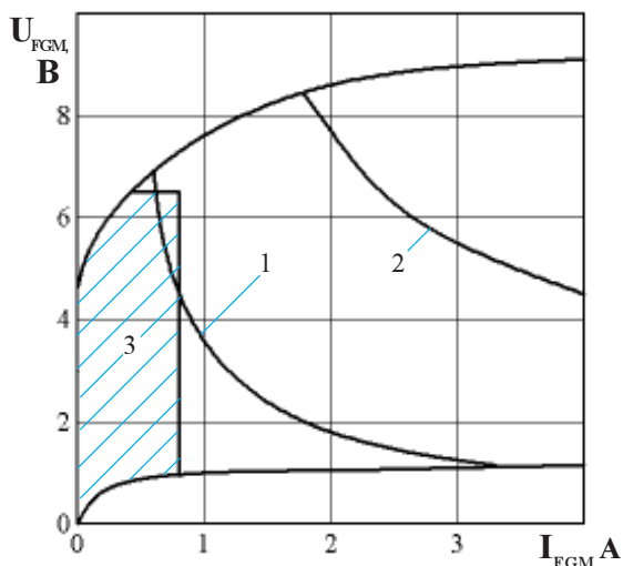
Рисунок 9 - Пределные характеристики цепи управления
