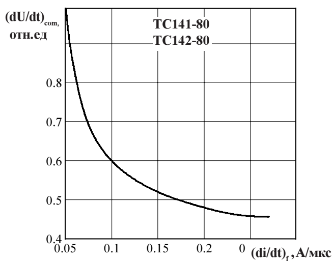
Рисунок 14 - Зависимость критической величины скорости нарастания коммутационного напряжения (dU/dt)_{com} от скорости спада предшествующего тока в открытом состоянии (di_T/dt)_f при амплитуде предшествующего тока в открытом состоянии I_T = I_{TRSM} и максимально допустимой температуре перехода T_{jm} .
