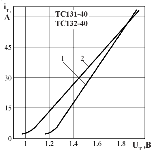
Рисунок 1 - Предельная вольтамперная характеристика в открытом состоянии при температуре перехода 25 °C (1) и максимальной температуре перехода T_{\text{jm}} (2)
