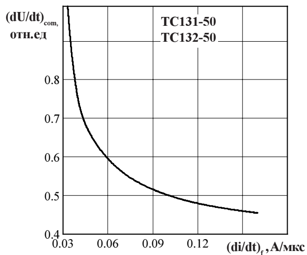
Рисунок 14 - Зависимость критической величины скорости нарастания коммутационного напряжения (dU/dt)_{com} от скорости спада предшествующего тока в открытом состоянии (di/dt)_f при амплитуде предшествующего тока в открытом состоянии I_T = I_{TRSM} и максимально допустимой температуре перехода T_{jm} .
