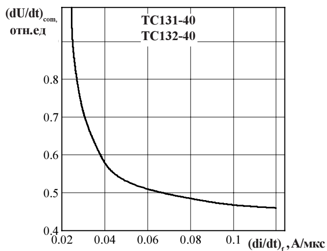
Рисунок 14 - Зависимость критической величины скорости нарастания коммутационного напряжения (dU/dt)_{com} от скорости спада предшествующего тока в открытом состоянии (di/dt)_f при амплитуде предшествующего тока в открытом состоянии I_T = I_{TRSM} и максимально допустимой температуре перехода T_{jm} .
