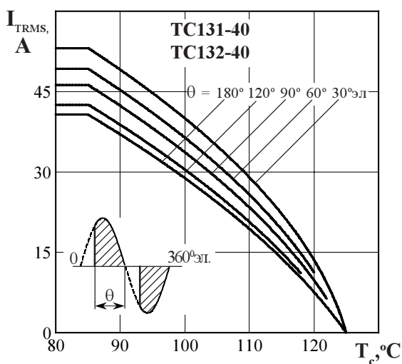
Рисунок 2 - Зависимость допустимого действующего тока в открытом состоянии I_{\text{TRMS}} от температуры корпуса T_c для токов синусоидальной формы частотой f = 50\text{ Гц}
