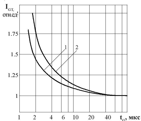
Рисунок 10 - Зависимость отпирающего импульсного тока управления I_{GT} от длительности управляющего импульса t_G при температуре перехода T_j = 25^\circ \text{C} (1), T_{jmin} = \text{минус } 50^\circ \text{C} (2) и напряжения в закрытом состоянии U_D = 12 \text{ В} .
