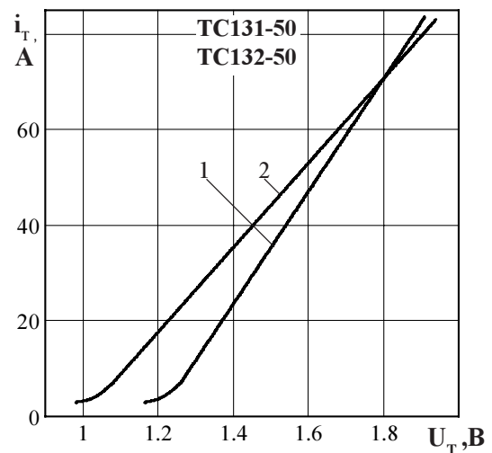
Рисунок 1 - Предельная вольтамперная характеристика в открытом состоянии при температуре перехода 25 °C (1) и максимальной температуре перехода T_{\text{jm}} (2)
