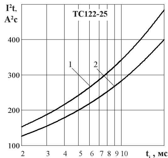
Рисунок 6 - Зависимость защитного показателя I^2t от длительности импульса тока t_i при исходной температуре структуры T_i = 25\text{ }^{\circ}\text{C} (1) и максимальной температуре T_{jm} (2)
