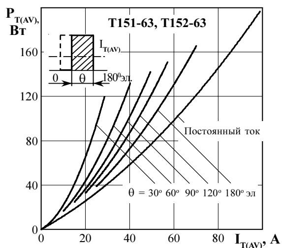
Рисунок 7 - Зависимость средней рассеиваемой мощности в открытом состоянии P_{T(AV)} от среднего тока в открытом состоянии I_{T(AV)} прямоугольной формы частоты f = 50 Гц и постоянного тока
