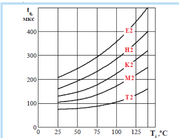
Рисунок 11 - Зависимость времени выключения t_q от температуры структуры T_j при I_1 = I_{TAVM} ; U_D = 0,67 U_{DRM} ; U_R = 100\text{ В} ; (di/dt)_f = 5\text{ А/мкс} ; dU_D/dt = 50\text{ В/мкс}
