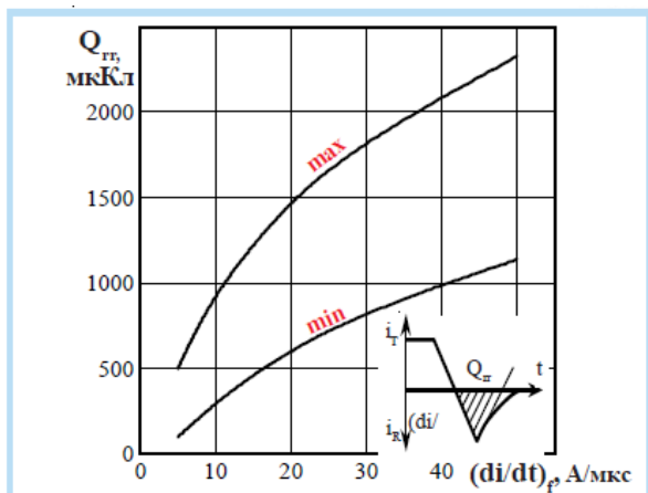
Рисунок 10 - Зависимость заряда восстановления Q_{rr} от скорости спада тока (di/dt)_f в открытом состоянии при T_{jm} = 140^\circ\text{C} ; U_R = 100\text{ В} ; I_1 = I_{TAVM} .
