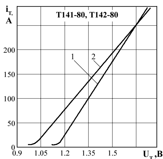
Рисунок 1 - Предельная вольтамперная характеристика в открытом состоянии при температуре перехода 25\text{ °C} (1) и максимальной температуре перехода T_{jm} (2) I_T = 3,14I_{T(AV)}
