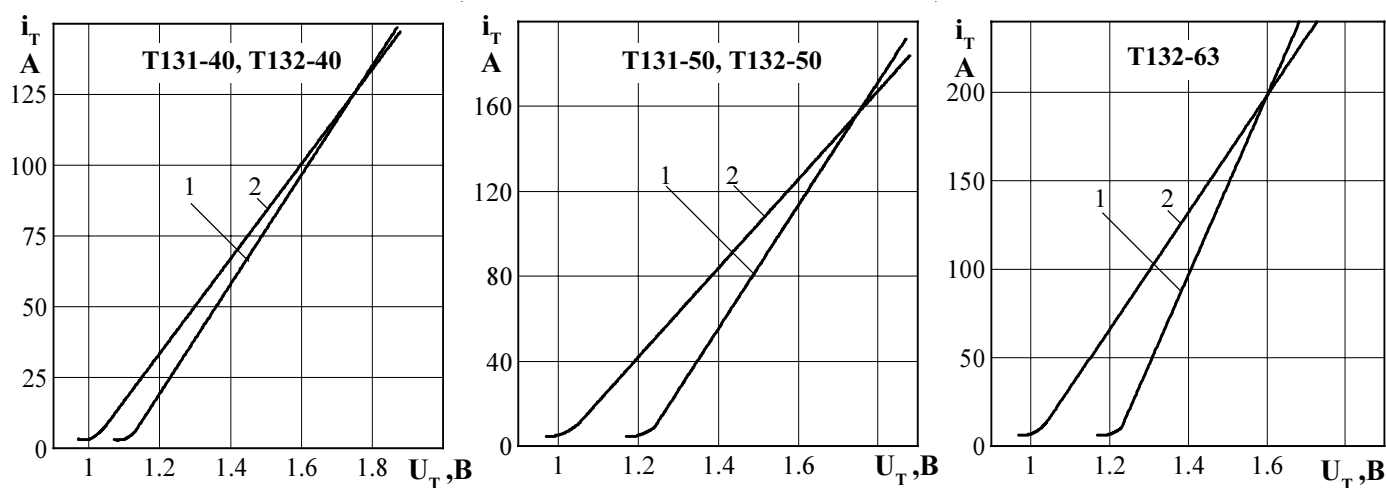
Рисунок 1 - Предельная вольтамперная характеристика в открытом состоянии при температуре перехода 25\text{ °C} (1) и максимальной температуре перехода T_{jm} (2) I_T = 3,14I_{T(AV)}
