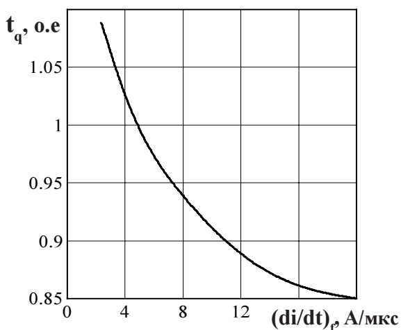
Рисунок 15 - Зависимость времени выключения t_q (о.е.) от скорости спада тока в открытом состоянии (di/dt)_f при T_{jm} = 125^\circ \text{C} ; I_T = I_{T(AV)} ; U_R = 100 \text{ В} ; dU_D/dt = 50 \text{ В/мкс} ; U_D = 0,67 U_{DRM}
