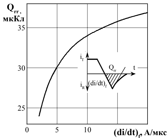
Рисунок 17 - Зависимость заряда восстановления Q_{rr} от скорости спада тока (di/dt)_p в открытом состоянии при температуре перехода T_{jm} = 125\text{ }^{\circ}\text{C} , U_{RM} = 100\text{ В} ; I_T = I_{T(AV)} .
