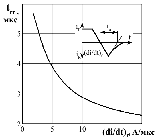
Рисунок 18 - Зависимость времени обратного восстановления t_{rr} от скорости спада тока (di/dt)_p в открытом состоянии при температуре перехода T_{jm} = 125\text{ }^{\circ}\text{C} , U_{RM} = 100\text{ В} ; I_T = I_{T(AV)} .
