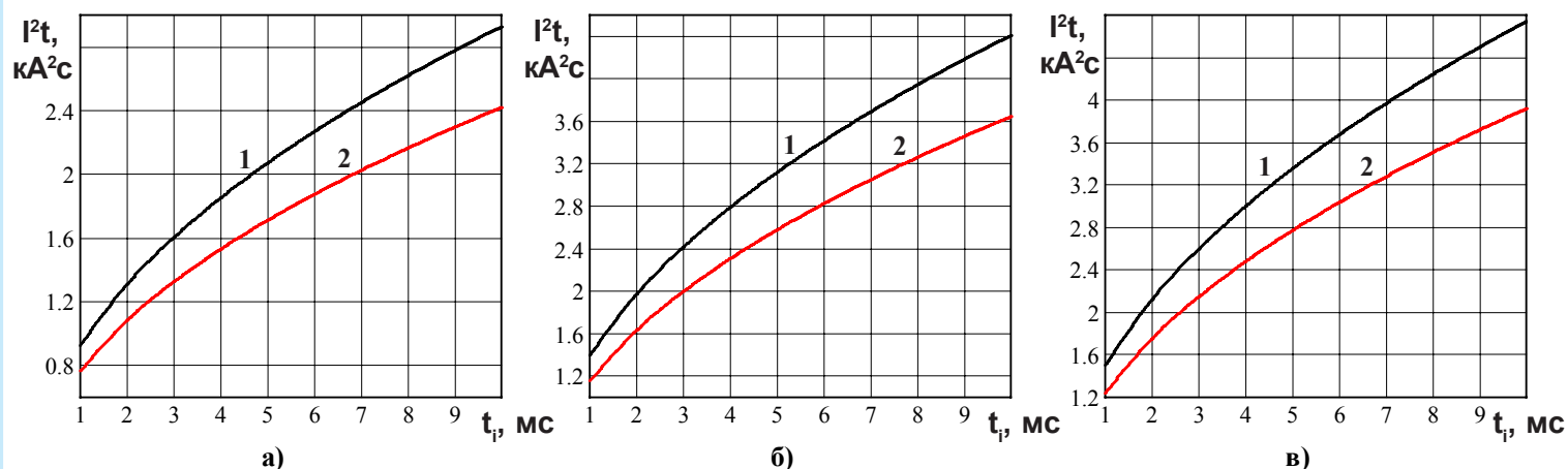
Рисунок 5 - Зависимость защитного показателя I^2t от длительности импульса тока t_i при температуре T_j = 25\text{ }^{\circ}\text{C} (1) и максимально допустимой температуре перехода T_{jm} (2) для модулей:
