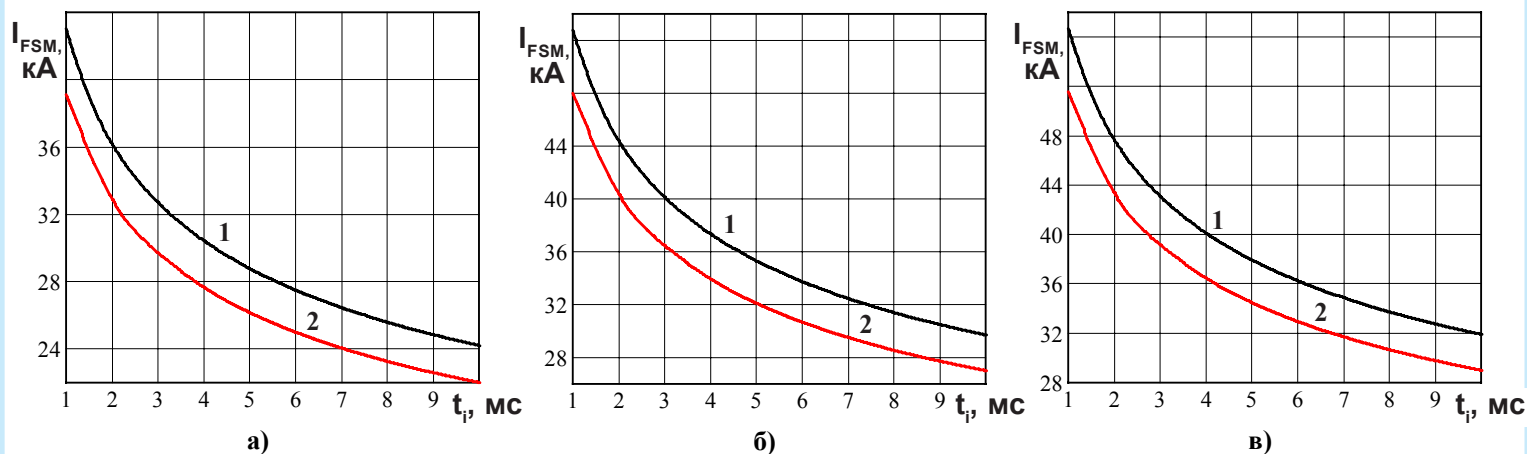
Рисунок 4 - Зависимость допустимой амплитуды ударного прямого тока I_{FSM} от длительности импульса тока t_p при исходной температуре структуры T_j = 25\text{ °C} (1) и максимально допустимой температуре перехода T_{jm} (2) для модулей:
