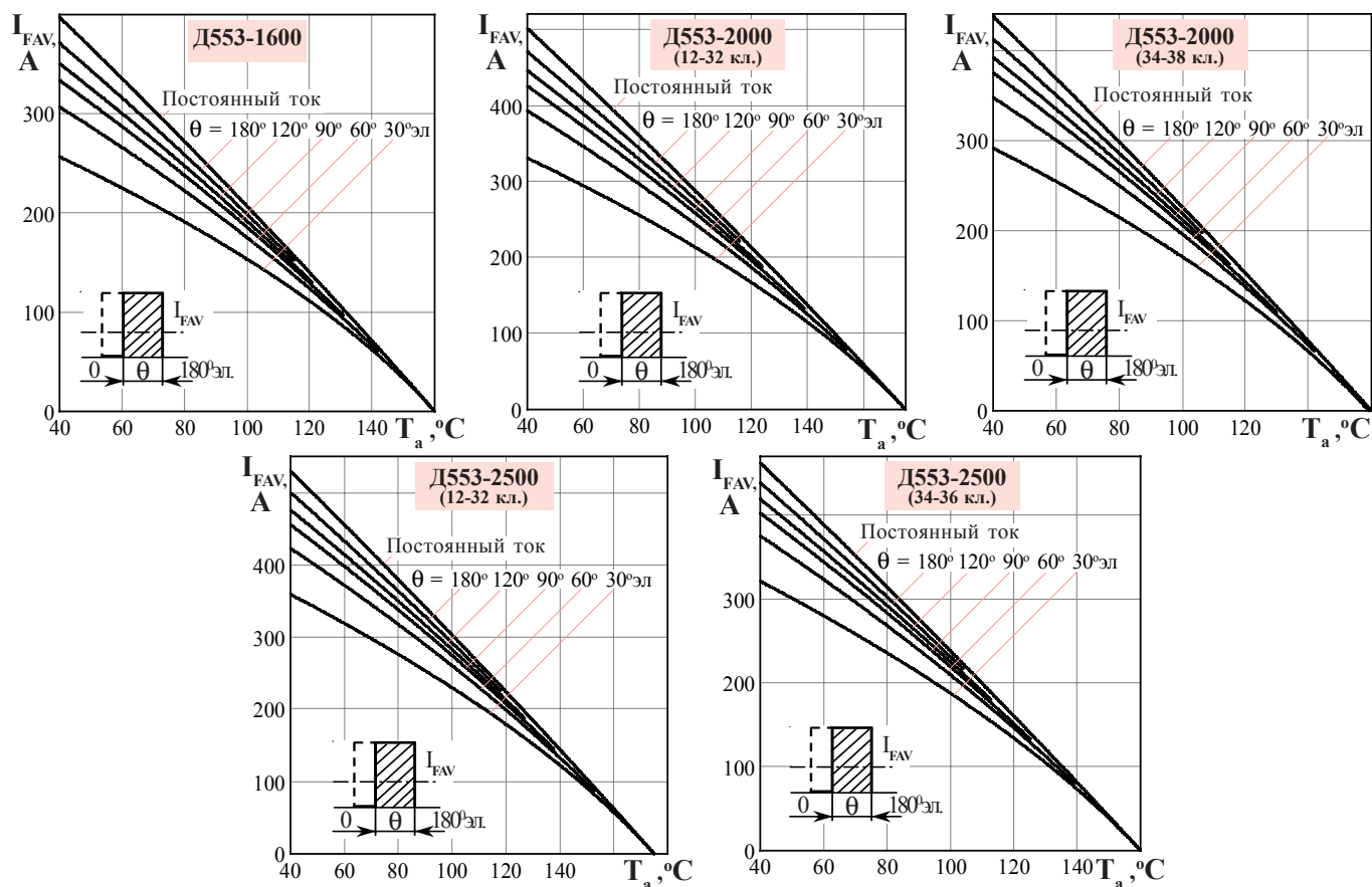
Рисунок 9 - Зависимость допустимого среднего прямого тока I_{FAV} от температуры окружающей среды T_a при естественном охлаждении на охлаждае ОР153-150 при различных углах проводимости для токов прямоугольной формы частотой f = 50 Гц и постоянного тока.
