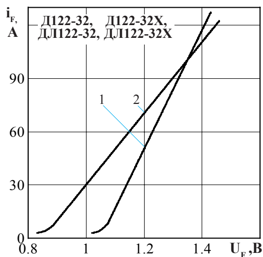
Рисунок 1 - Предельная прямая вольтамперная характеристика при температуре перехода 25 °C (1) и максимальной температуре перехода T_{jm} (2) I_F = 3, 14 I_{F(AV)}
