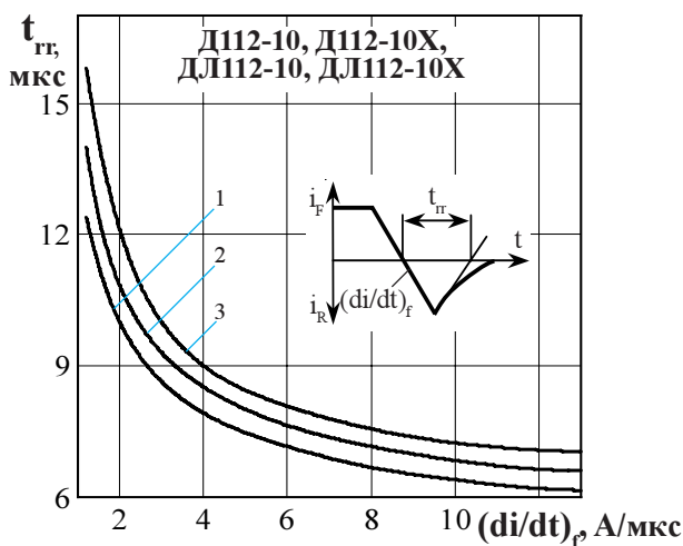
Рисунок 15 - Зависимость времени обратного восстановления t_{гр}
