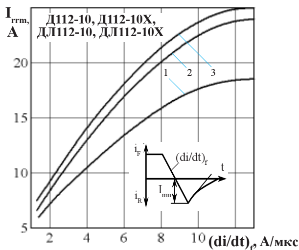
Рисунок 16 - Зависимость обратного тока восстановления I_{грm}
