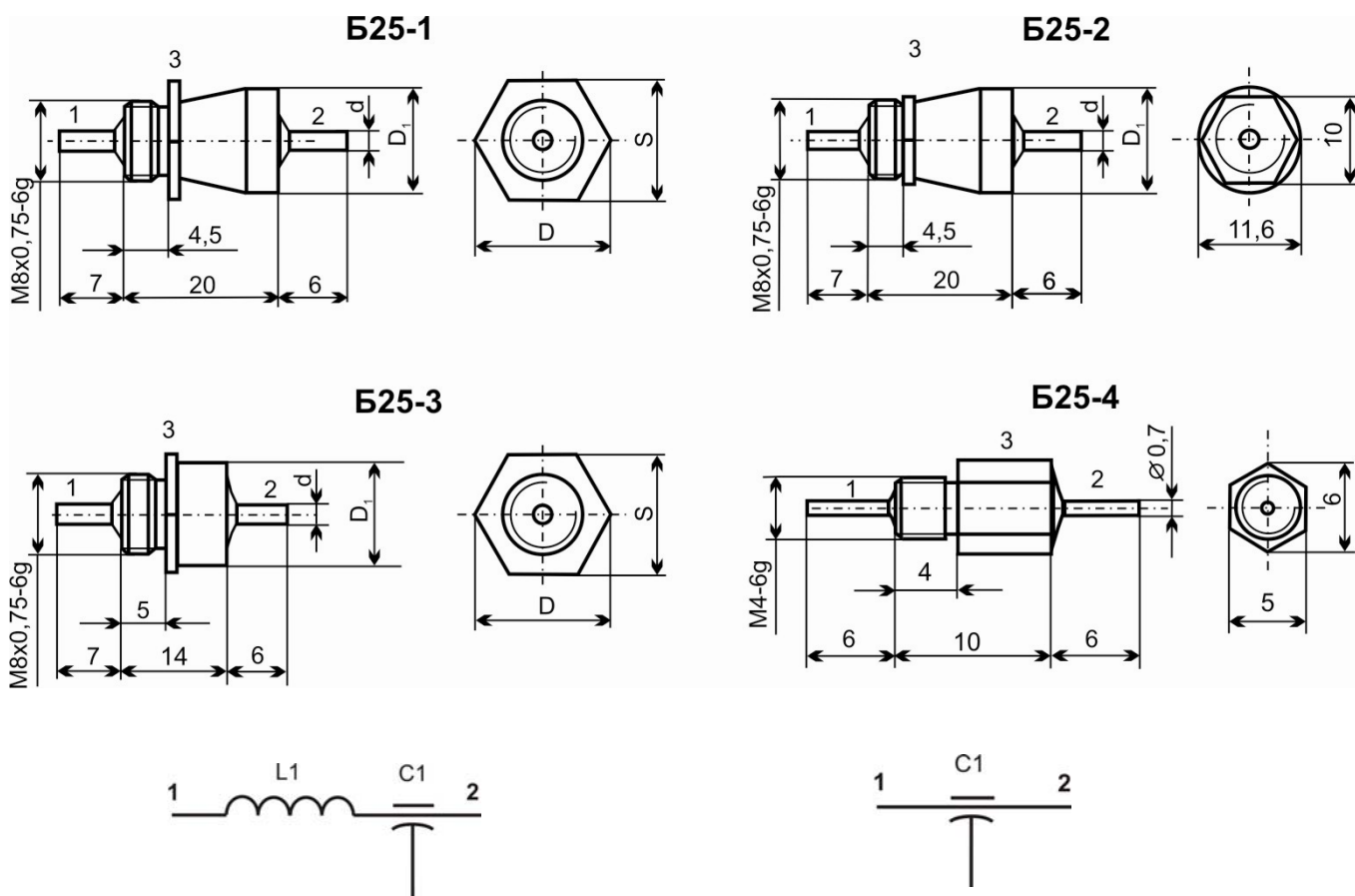
Схема электрическая фильтров Б25-1, Б25-2 с I_{\text{НОМ}} = 25 \text{ А} ; фильтров Б25-3 с I_{\text{НОМ}} = 10 \text{ А} и 25 \text{ А} ; фильтров Б25-4 с I_{\text{НОМ}} = 10 \text{ А} .
